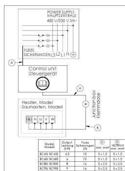
3-phase electrical connections of control unit C150 and BC-E heater 3-phasescher Elektroanschluss des Steuergeräts C150 und des Saunaofens BC-E
